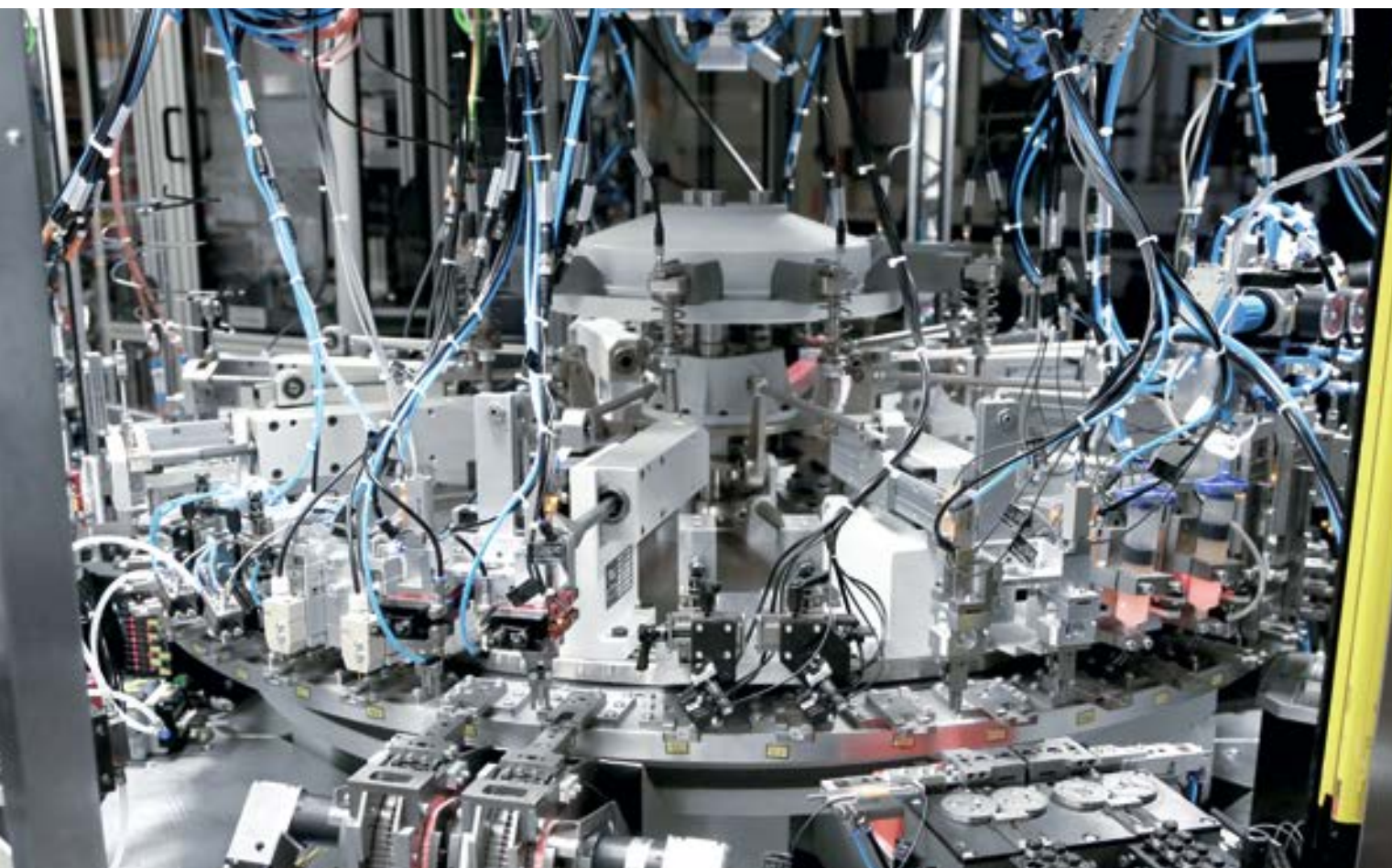
Assembly of small parts at Hammermeister Sondermaschinenentwicklung GmbH
